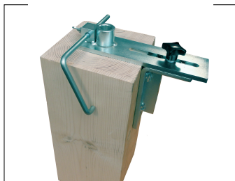
50020.3000 Bohrlehre Ø 30 mm
