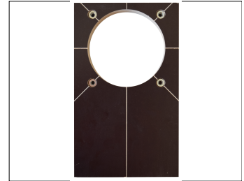
58000.1100 Frässhablone für FM8 (Art. Nr. 58000.0000) zum auffräsen Ø 100 mm
